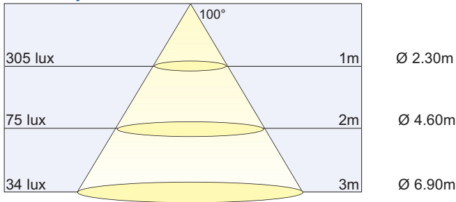
Natuurlijk wit 4000K 900LM
