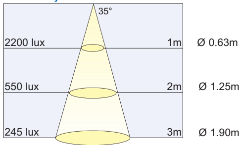
Natuurlijk wit 4000K 720LM
