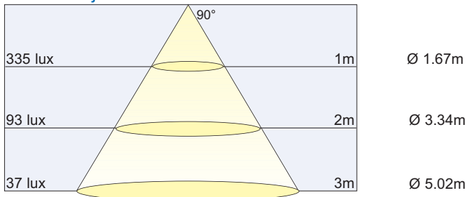
Natuurlijk wit 4000K 1800LM
