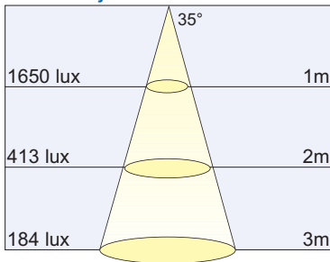
Natuurlijk wit 3800K 550LM
