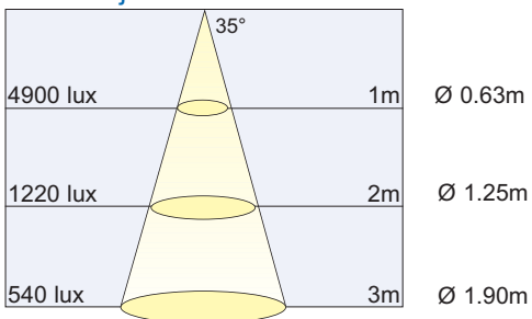
Natuurlijk wit 4000K 1560LM
