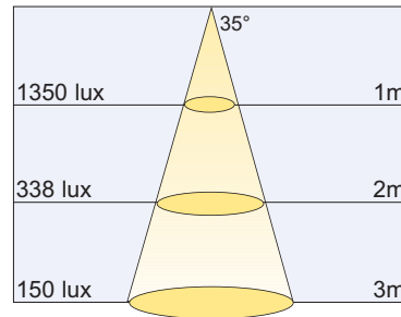
Warm wit 2800K 450LM
