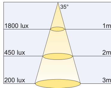
Warm wit 2800K 600LM
